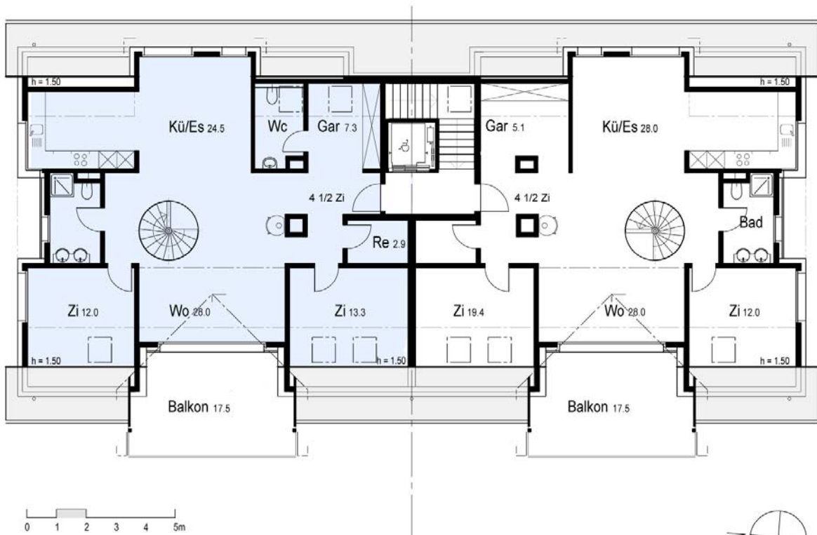
1. Dachgeschoss
