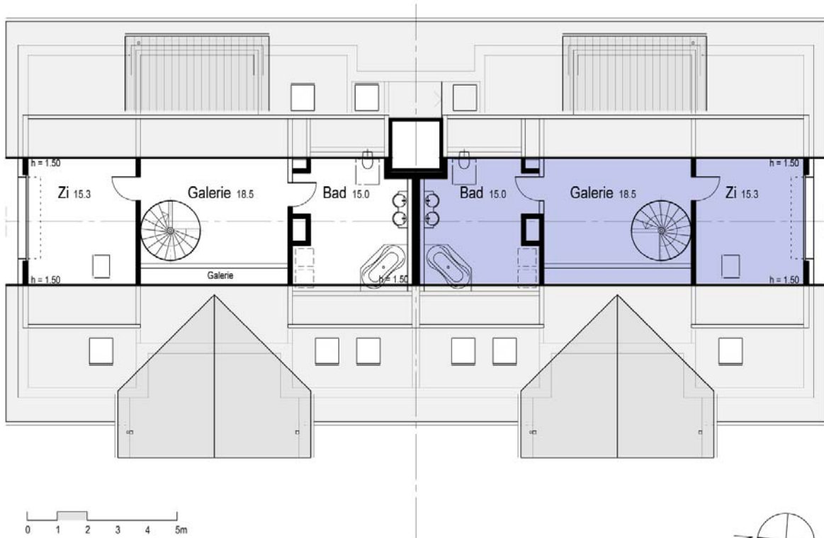
2. Dachgeschoss
